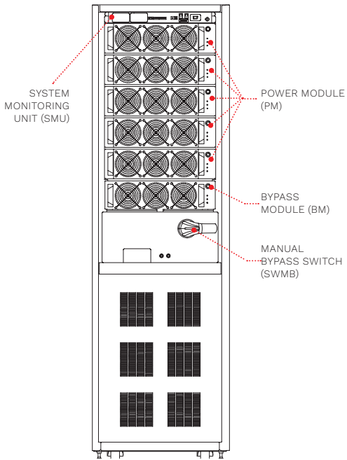
Avec bypass manuel jusqu'à 300 kW
