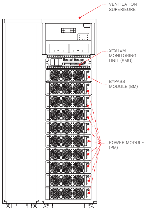
MP2 600 PCO VE* (avant)
